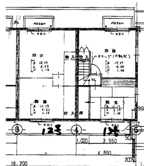
2階平面図 131.0
